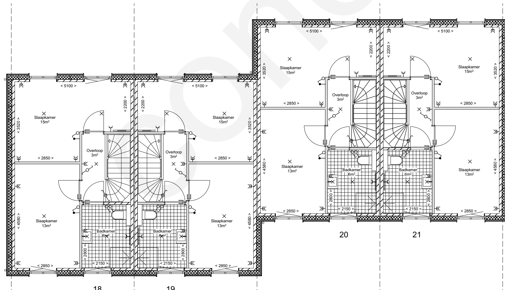
1E VERDIEPING
