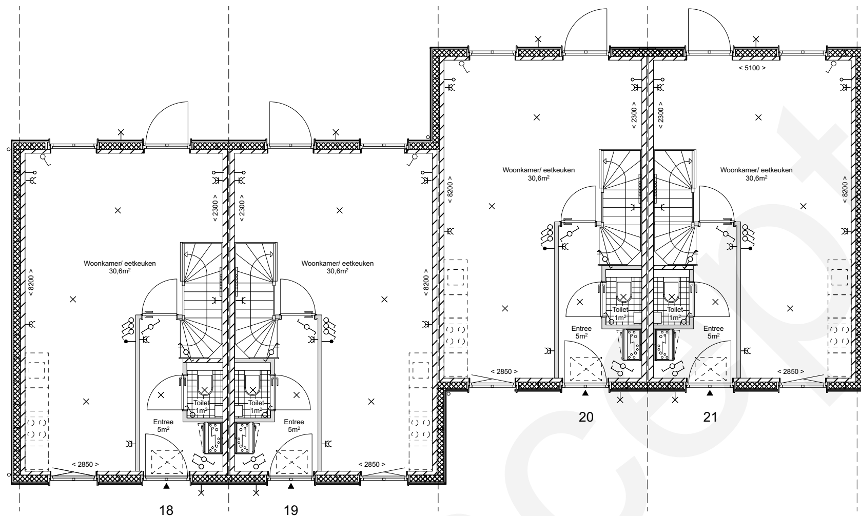
BEGANE GROND
