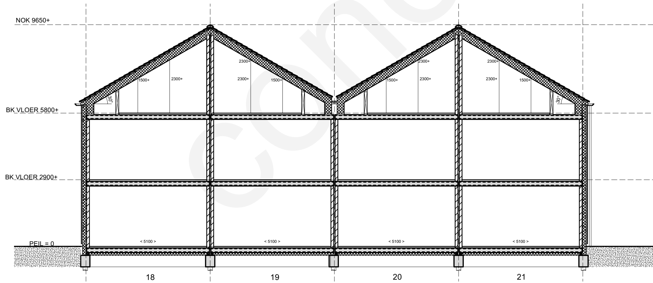
DOORSNEDE
