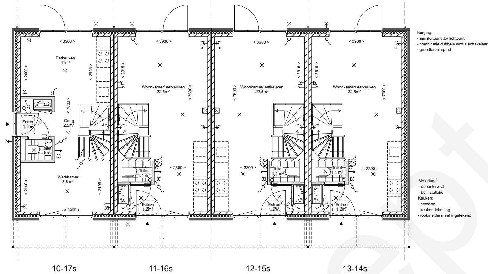
BEGANE GROND
