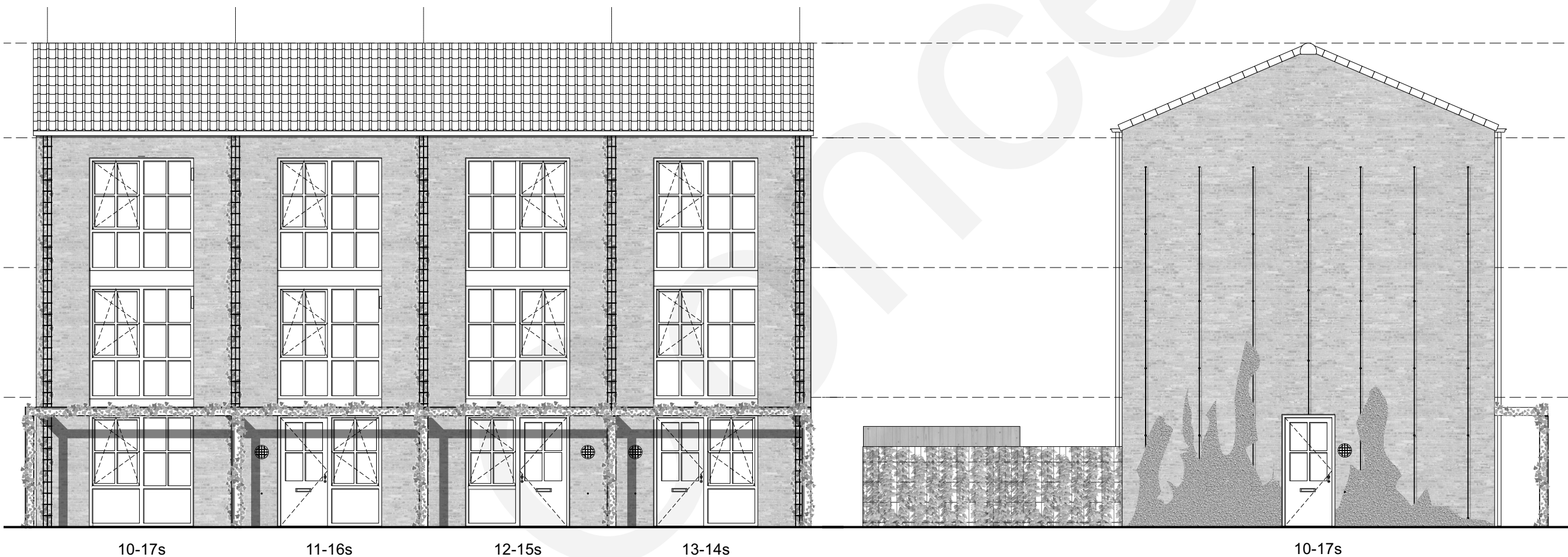
ZIJGEVEL
