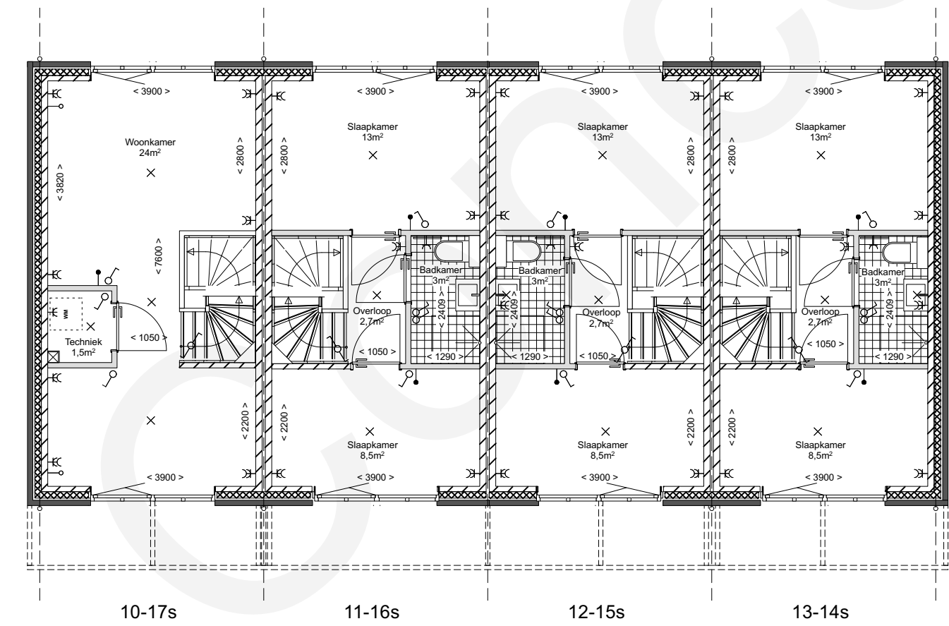
1E VERDIEPING
