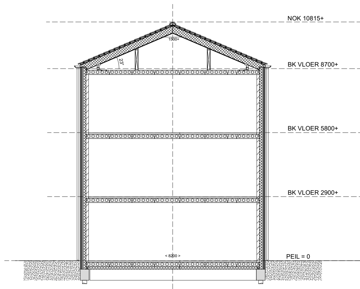
DOORSNEDE
