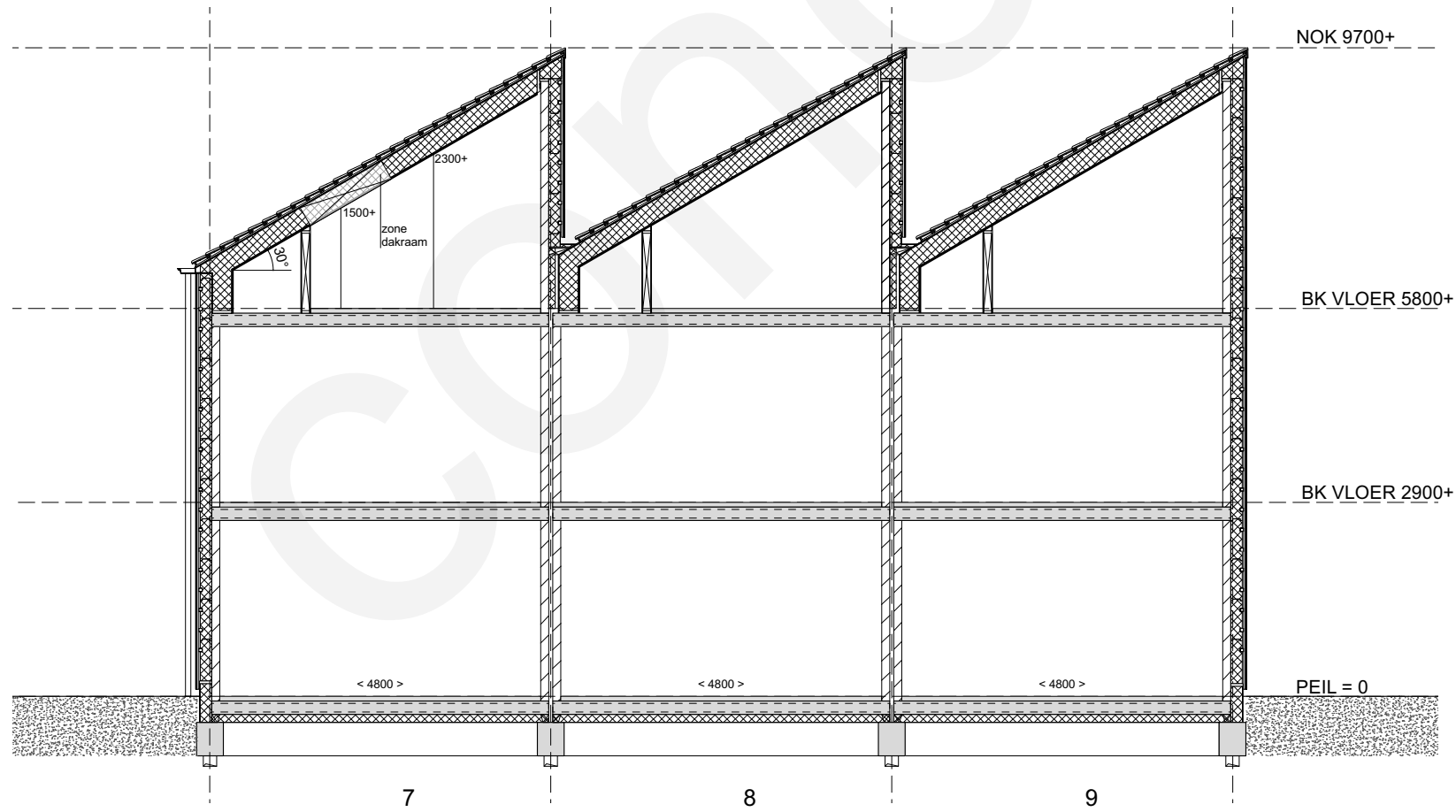
DOORSNEDE
