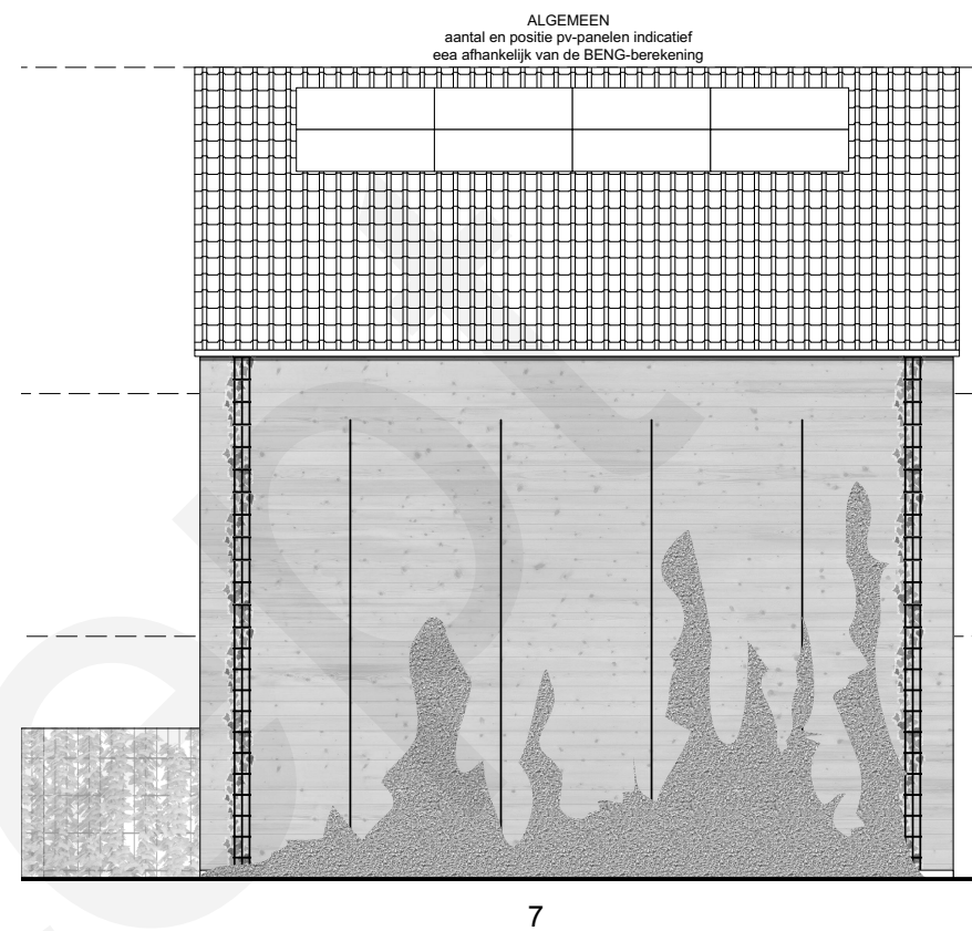
ZIJGEVEL
