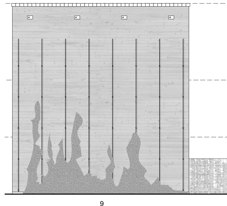
ZIJGEVEL
