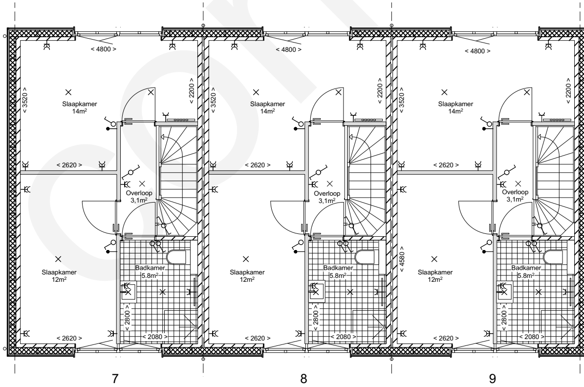
1E VERDIEPING
