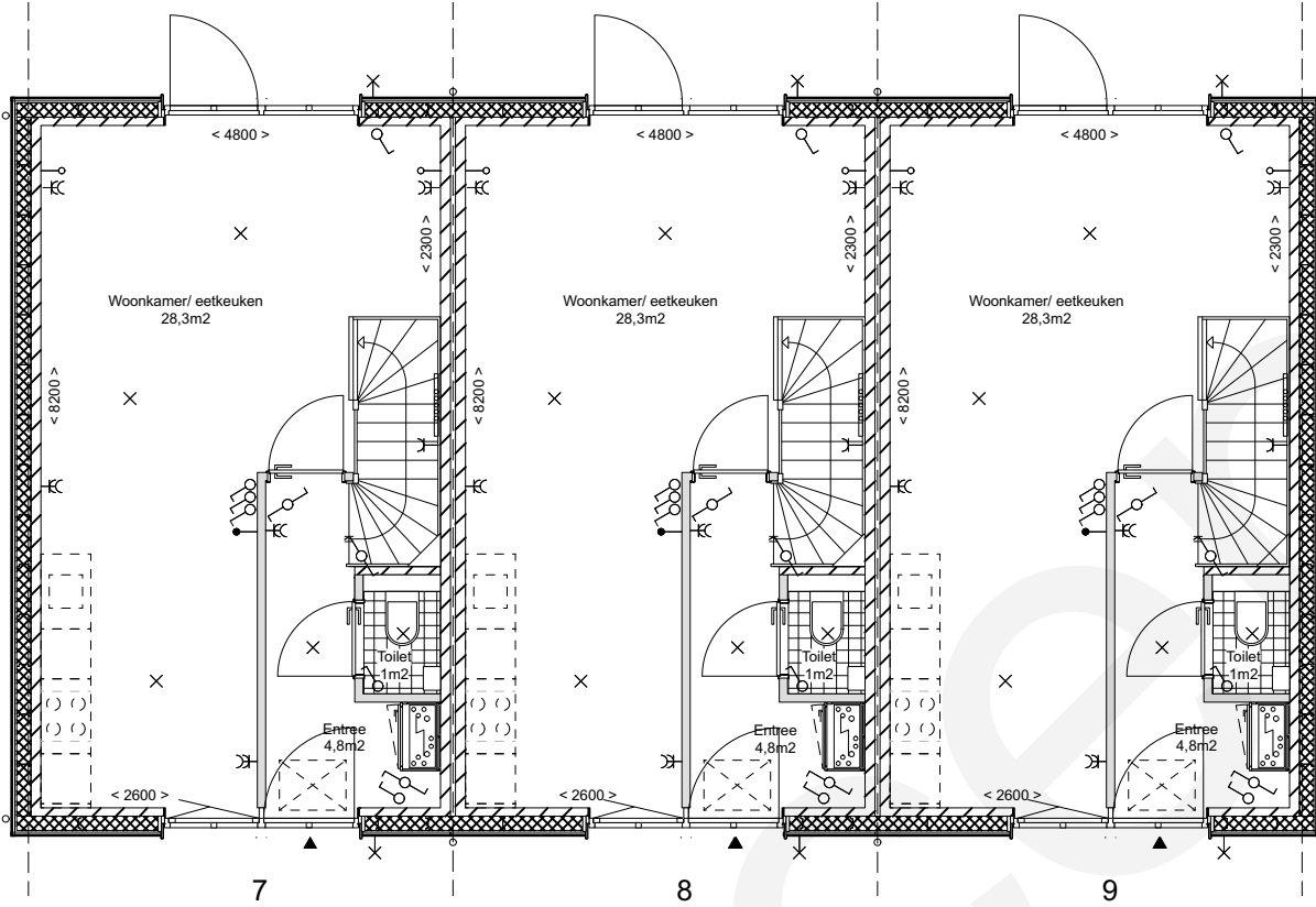
BEGANE GROND
