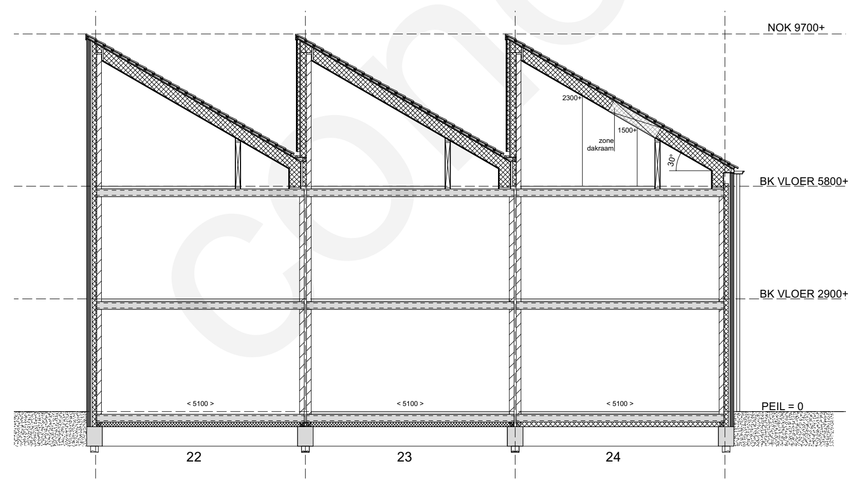
DOORSNEDE
