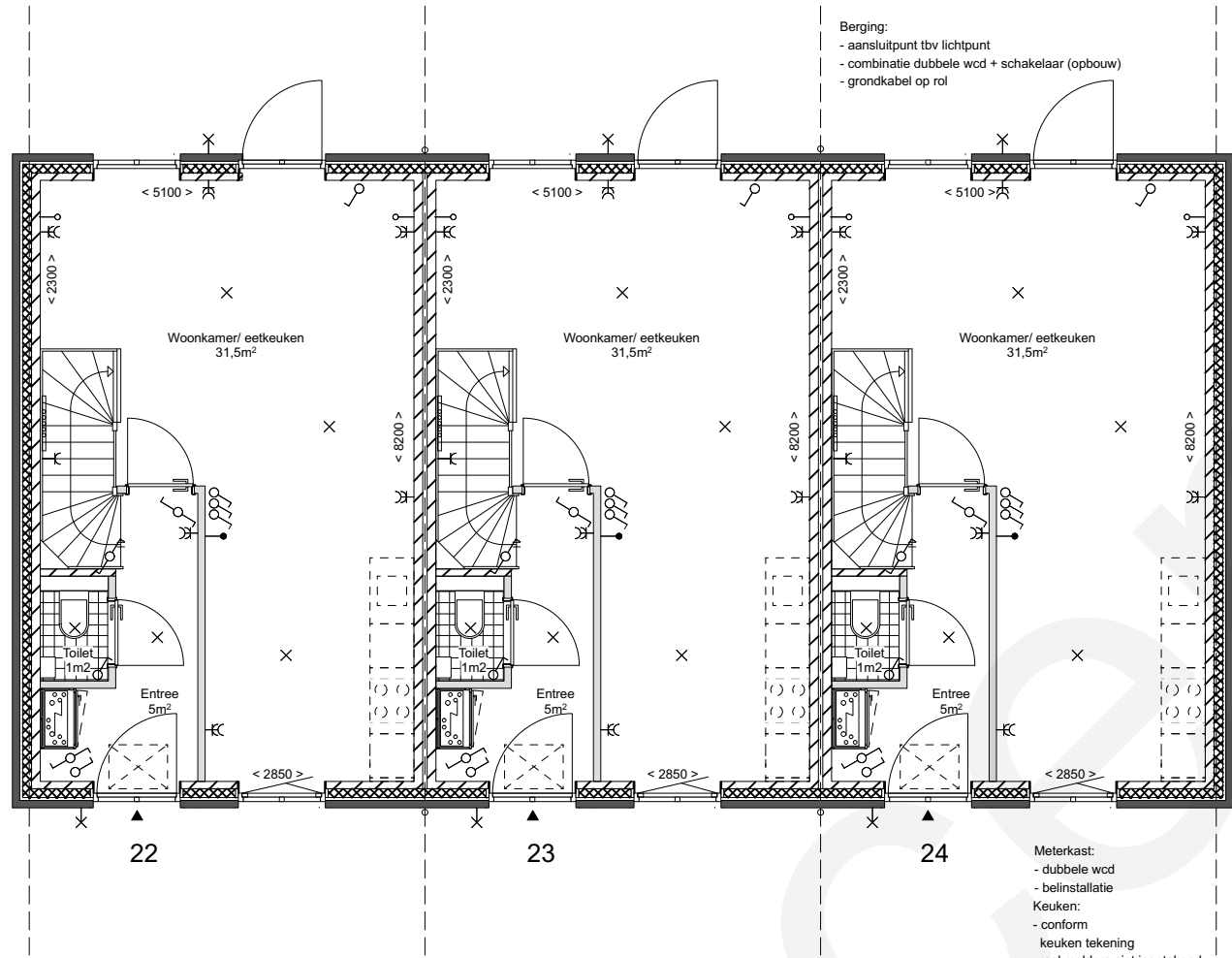
BEGANE GROND
