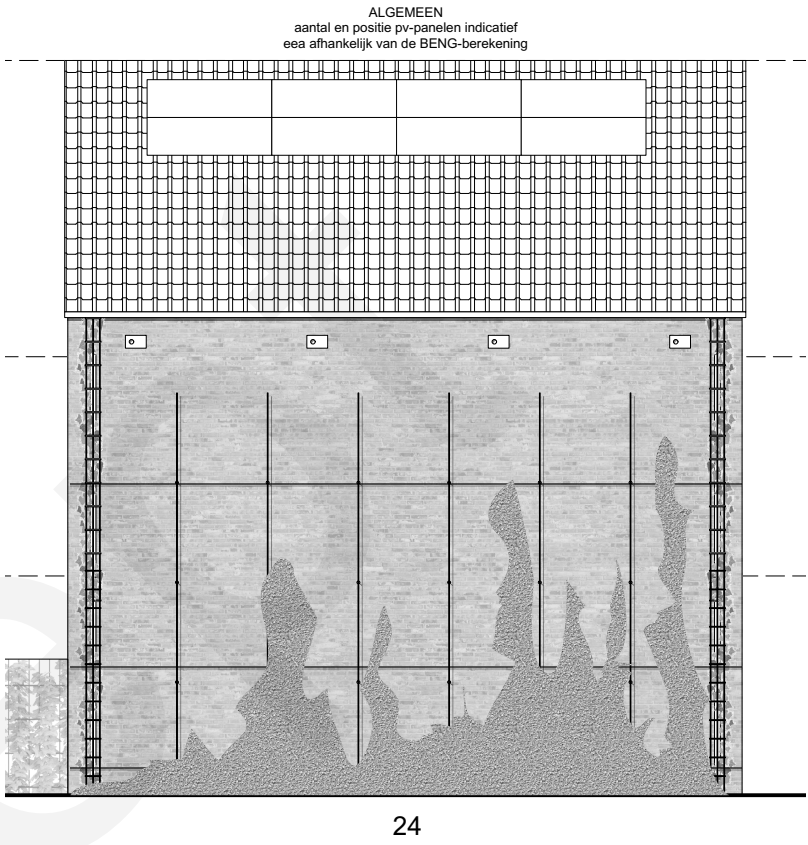
ZIJGEVEL
