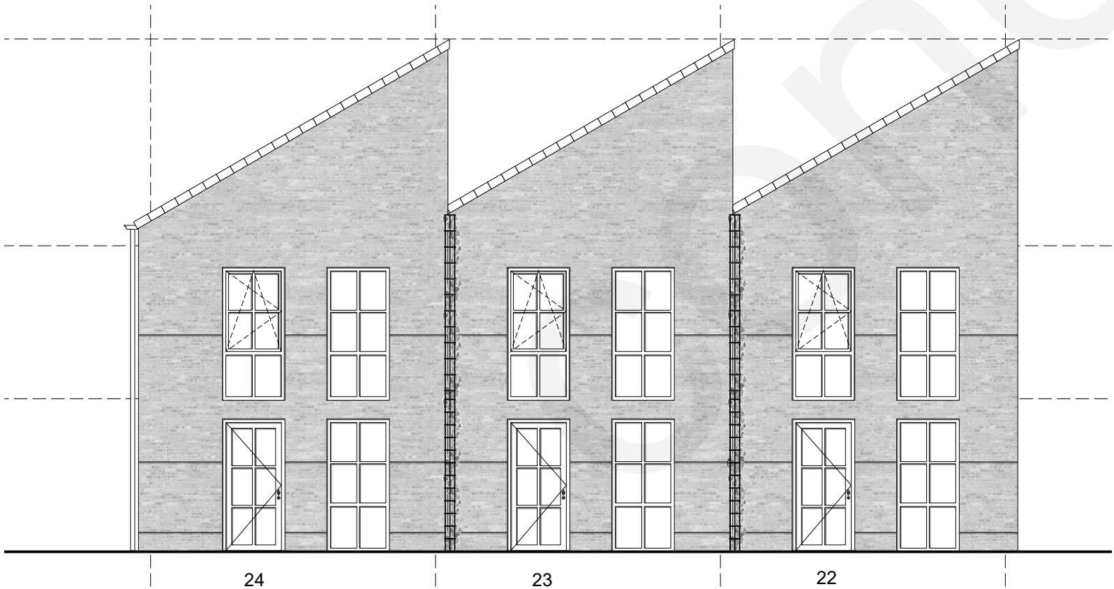
ACHTERGEVEL
