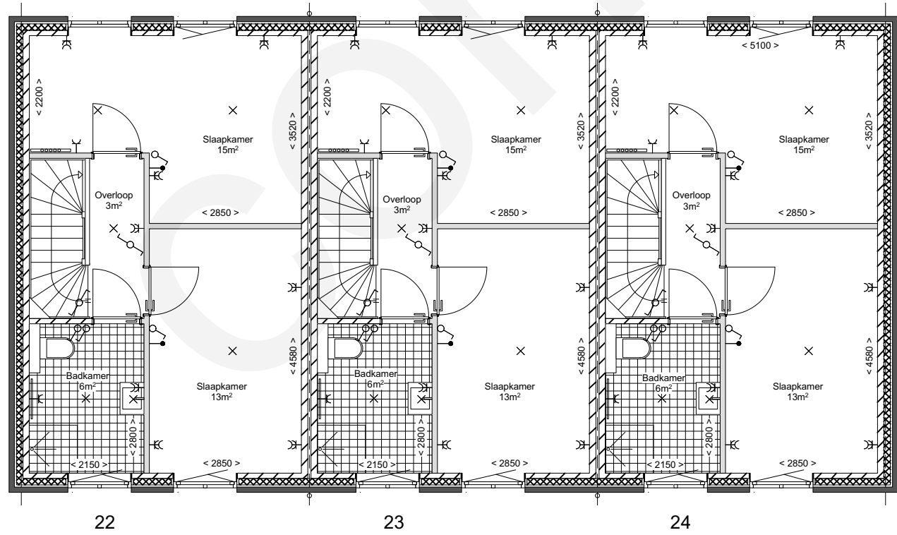
1E VERDIEPING
